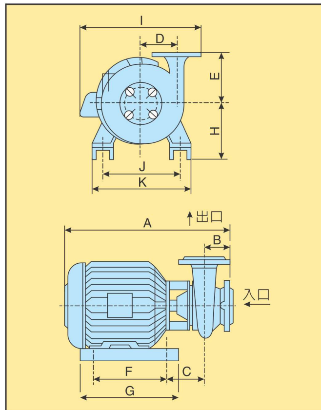
4P(4極)三相外觀尺寸圖 (50Hz(1450R.P.M.))
